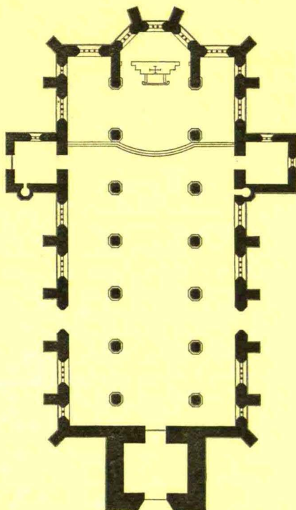
Abb. 117. Grundriß der Lambertikirche auf der Neustadt Hildesheim.
