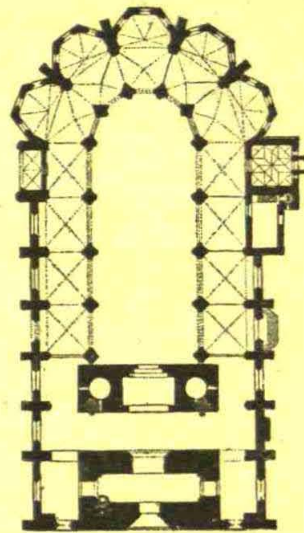
Abb. 98. Grundriß der Andreaskirche in Gildesheim.
